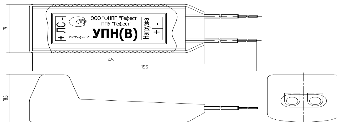
Рисунок 1 Внешний вид устройства (для УПН(С) надпись на корпусе соответственно «УПН(С)»)
