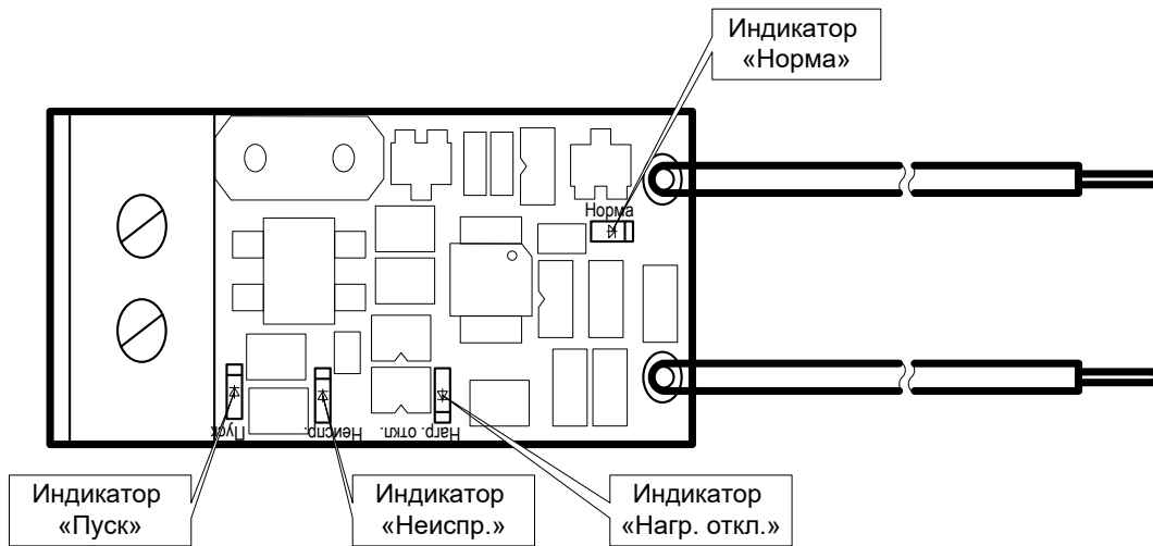
Рисунок 4 Расположение светодиодов
